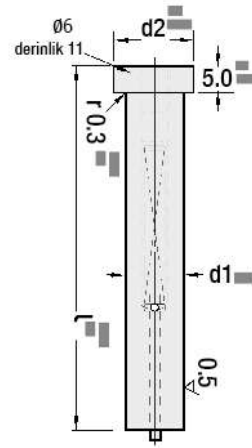
ISO 8020 Merkezleme Pimli - İtici, Zimba
