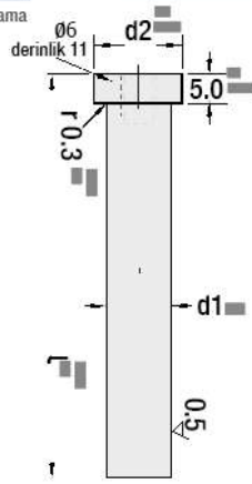
ISO 8020 Merkezleme Pimli - Zimba
